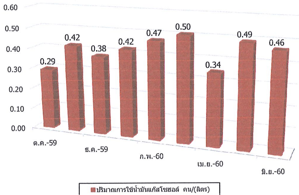
ปริมาณการใช้น้ำมันแก๊สโซฮอล์ 91 คน/(ลิตร) อาคารสำนักงานอธิการบดี
