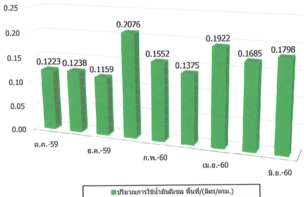
ปริมาณการใช้น้ำมันดีเซล พื้นที่(ลิตร/ตรม.) อาคารสำนักงานอธิการบดี
