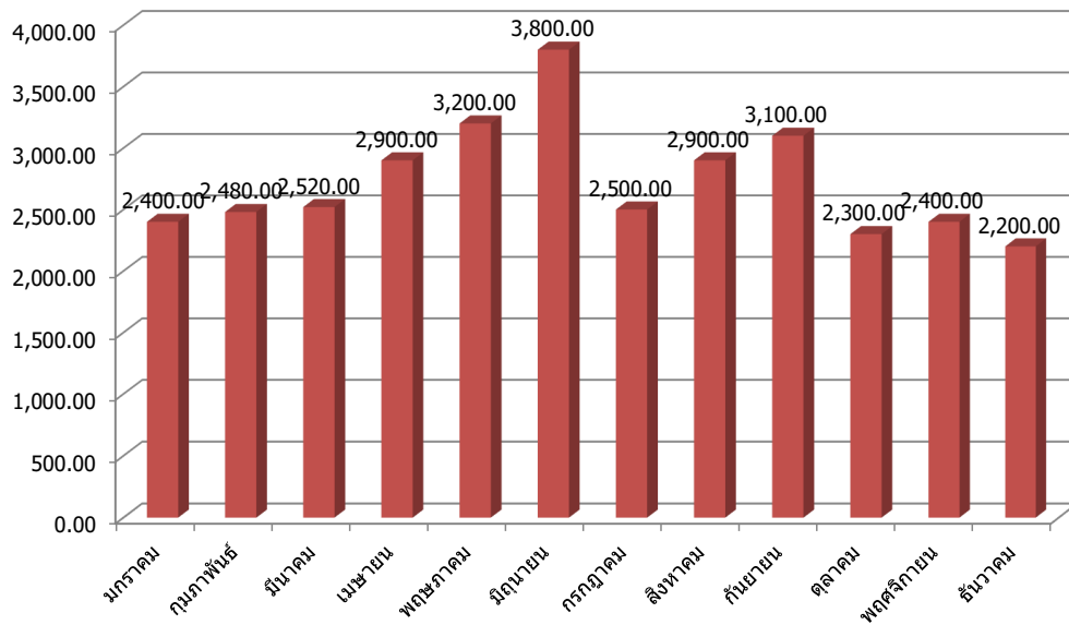
ปริมาณการใช้ไฟฟ้า (kWh) ประจำปี 2560
