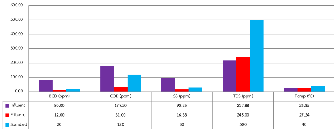
ค่าเฉลี่ยคุณภาพน้ำ โรงบำบัดน้ำเสียรวม มหาวิทยาลัยแม่โจ้ (ธันวาคม 2564)
