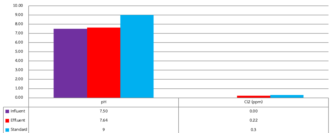
ค่าเฉลี่ยคุณภาพน้ำ โรงบำบัดน้ำเสียรวม มหาวิทยาลัยแม่โจ้ (ธันวาคม 2564 )
